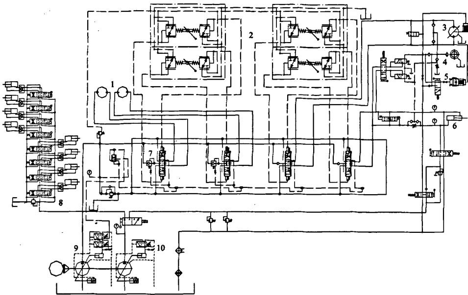
图2 ZDY6000L型履带式全液压坑道钻机液压系统原理图
