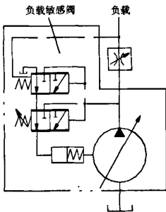
图 1 负载敏感控制原理图
